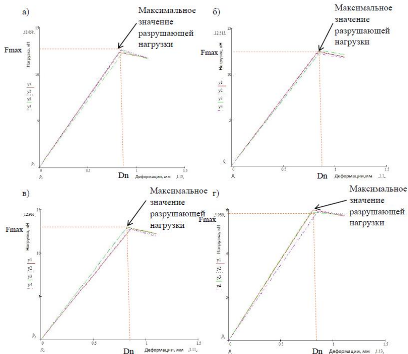
Рисунок 5 – Результаты испытаний механической связи в виде однонаправленной углеродволоконной ленты замкнутого контура. Графики зависимости полных средних деформаций по четырем образцам от прилагаемой нагрузки для каждого типа двухсрезного образца: а – тип 1; б – тип 2; в – тип 3; г – тип 4
