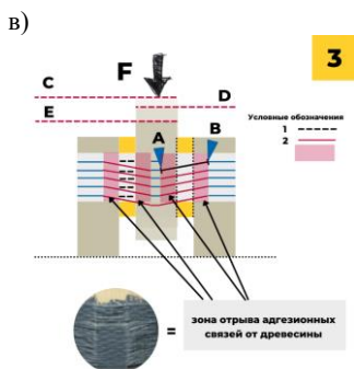
Рисунок 7 – Механизм разрушения механической связи в виде однонаправленной углеродоволоконной ленты замкнутого контура: a – этап до приложения нагрузки; б – этап приложения нагрузки; в – этап после приложения разрушающей нагрузки
