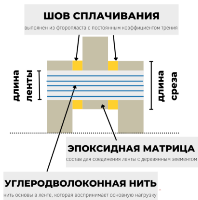
Рисунок 3 – Конструкция двухсрезного образца с механической связью в виде однонаправленной углеродоволоконной ленты в виде замкнутого контура с указанием длин для определения коэффициента армирования
