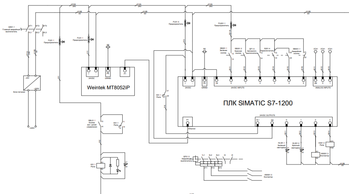
Рис.2. Принципиальная схема шкафа управления.
