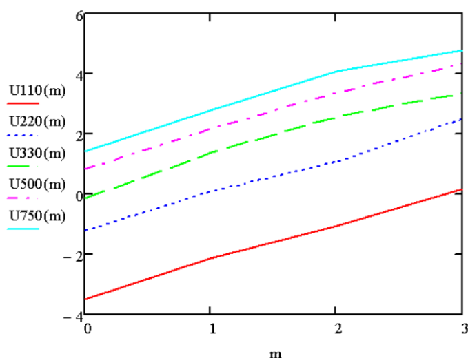
Рис.1. Логарифмический график удельных потерь мощности на корону, где 0–хорошая погода, 1–сухой снег, 2–дождь, 3–изморозь.
