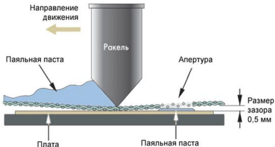
Рис.1. Нанесение паяльных паст методом трафаретной печати.
