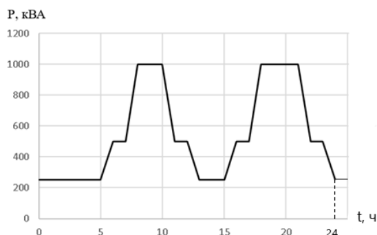
Рис.2. Суточная нагрузочная диаграмма работы трансформатора.
