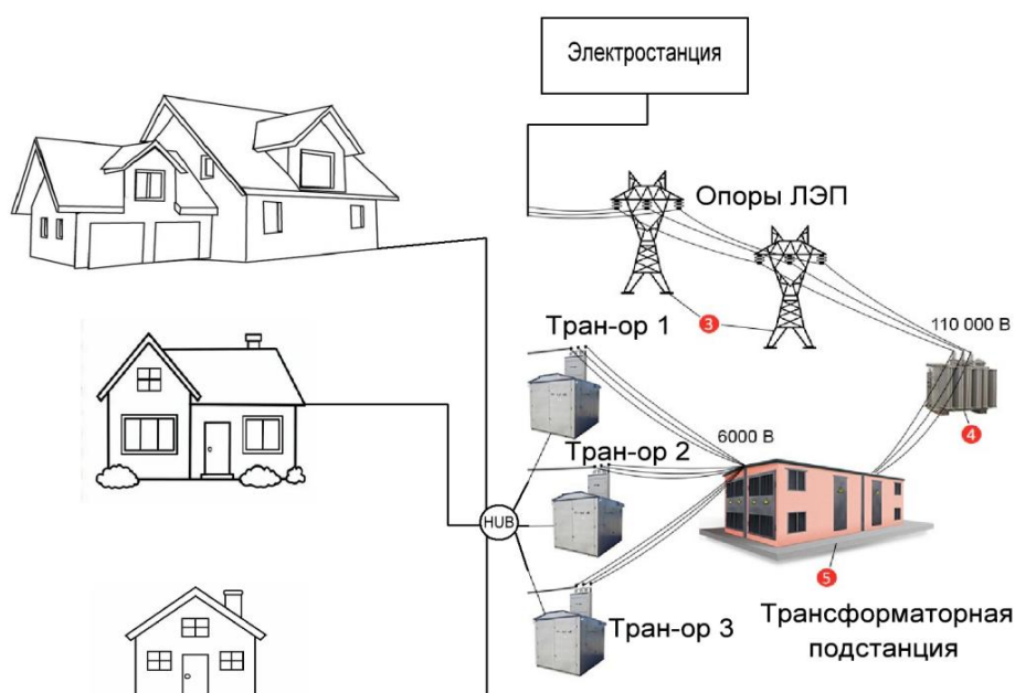
Рис.1. Пространственное размещение элементов на трансформаторной станции.
