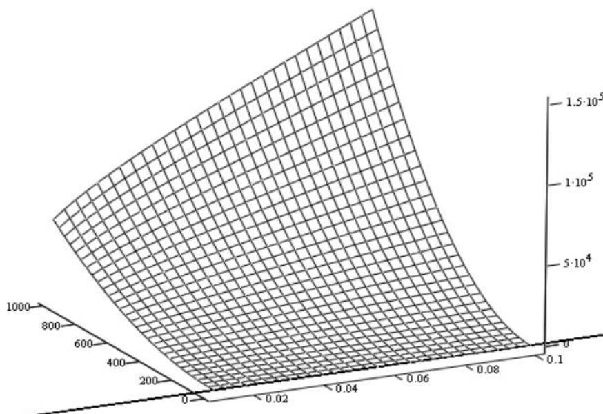
Рис.3. Пространственный график зависимости потерь мощности(Вт) от напряжения в линиях(кВ) и радиуса проводника(м).
