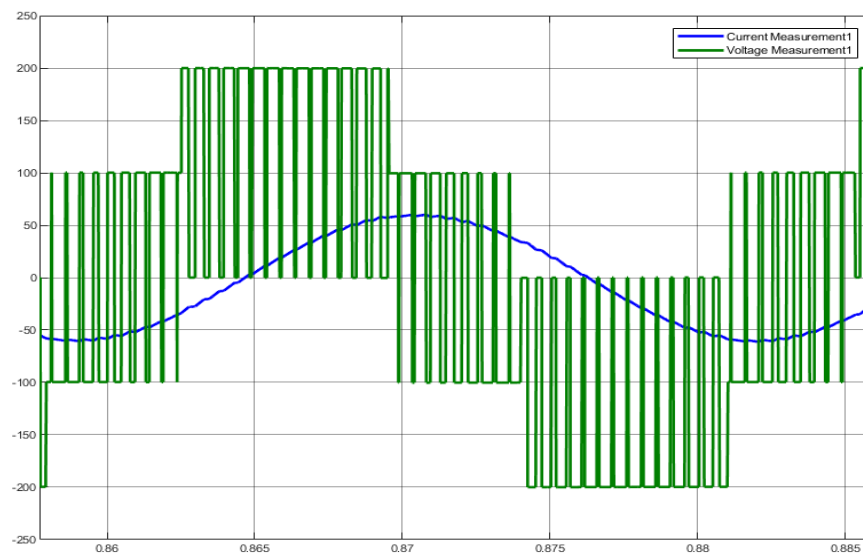
Рис.3. Графики тока (синий) и напряжения (зеленый).
