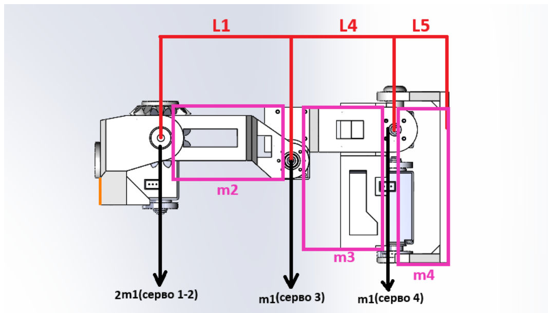
Рис.2. Схематичное изображение манипулятора ноги.
