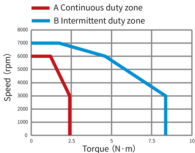
Рис.3. График зависимости момента от скорости синхронного двигателя с постоянными магнитами.
