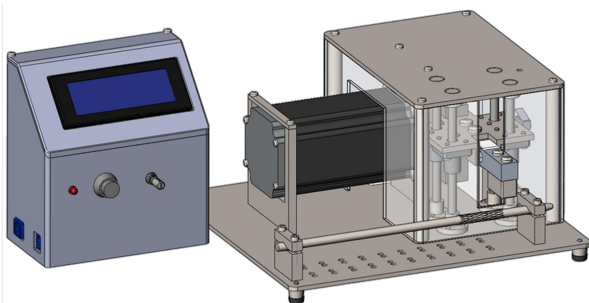
Рис.2. Конструкция автоматической установки.
