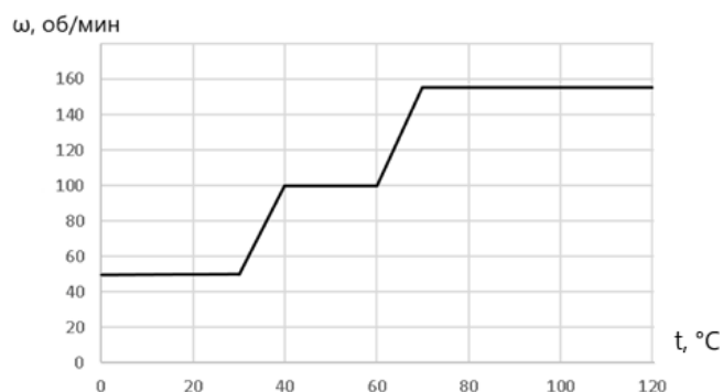
Рис.1. Зависимость скорости вращения вентилятора от температуры.
