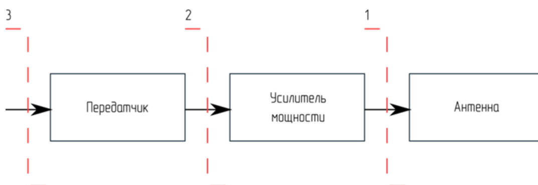
Рис.1. Способы размещения вращающегося перехода.
