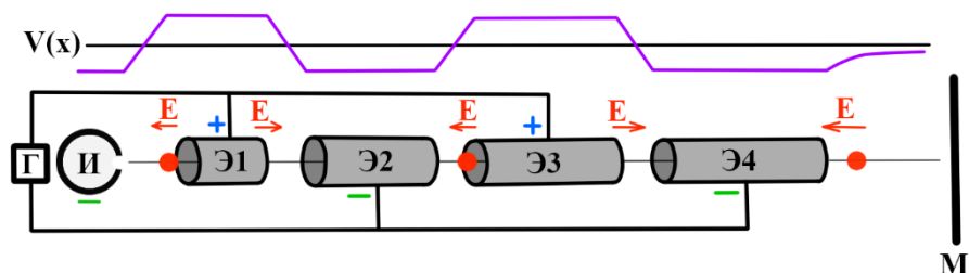
Рис.1. Принцип работы линейного ускорителя:
