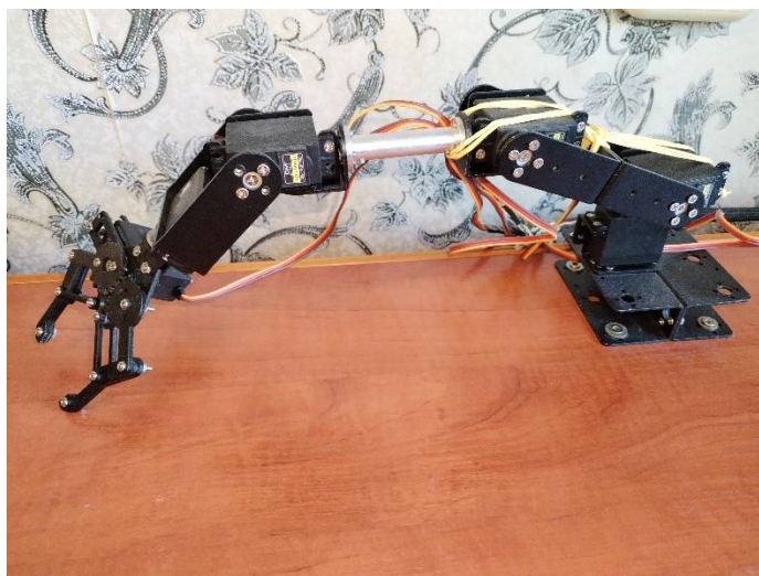
Рис.1. Внешний вид робота-манипулятора.
