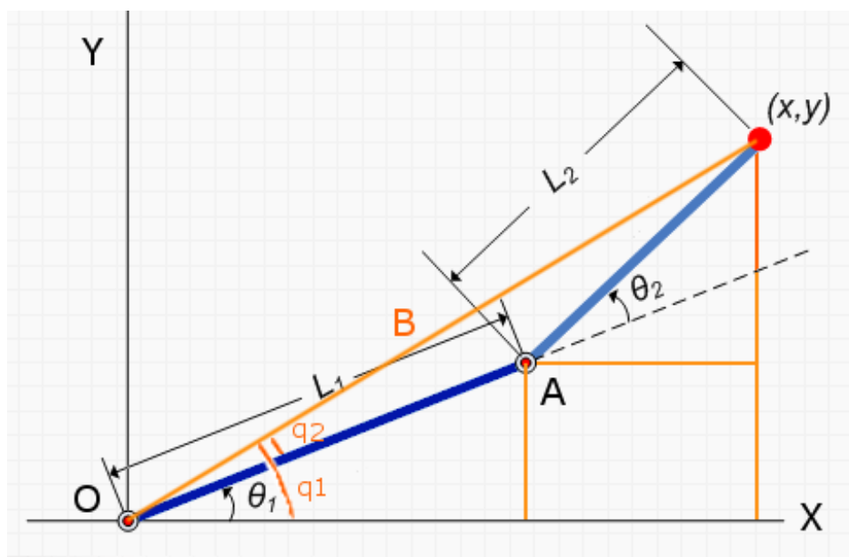
Рис.1. Решение обратной задачи кинематики.
