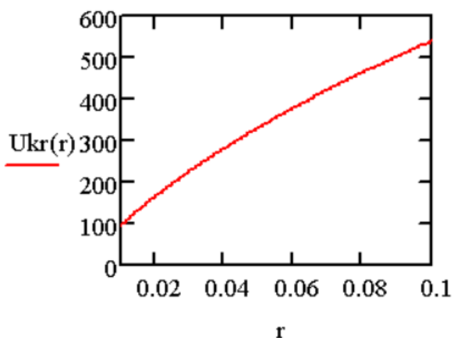
Рис.2. График зависимости критического напряжения от радиуса проводника.
