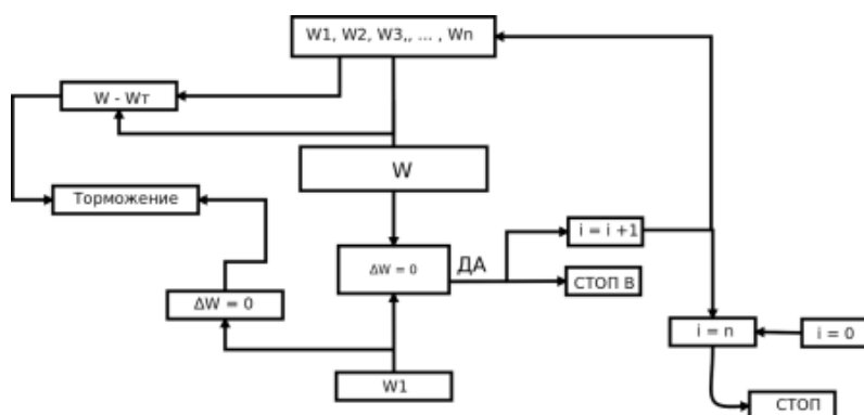
Рис.1. Блок-схема управления процессом торможения.
