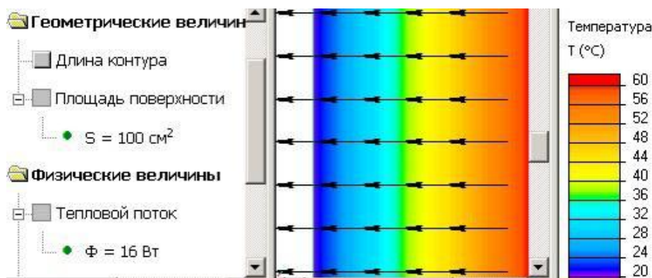
Рис.1. Закон Фурье.
