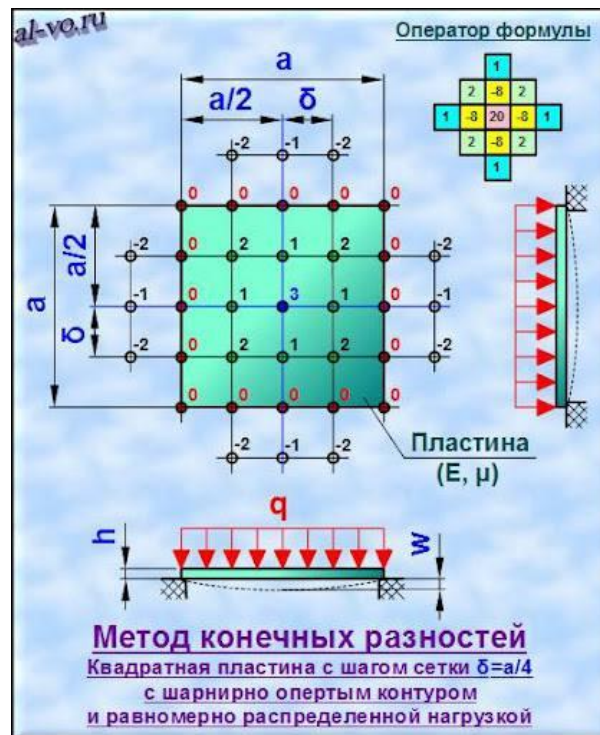
Рис.4. Метод конечных разностей.
