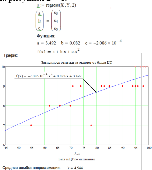
Рис.16. Квадратичная регрессия.
