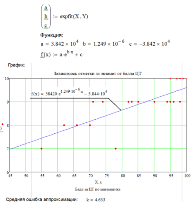
Рис.5. Экспоненциальная регрессия.
