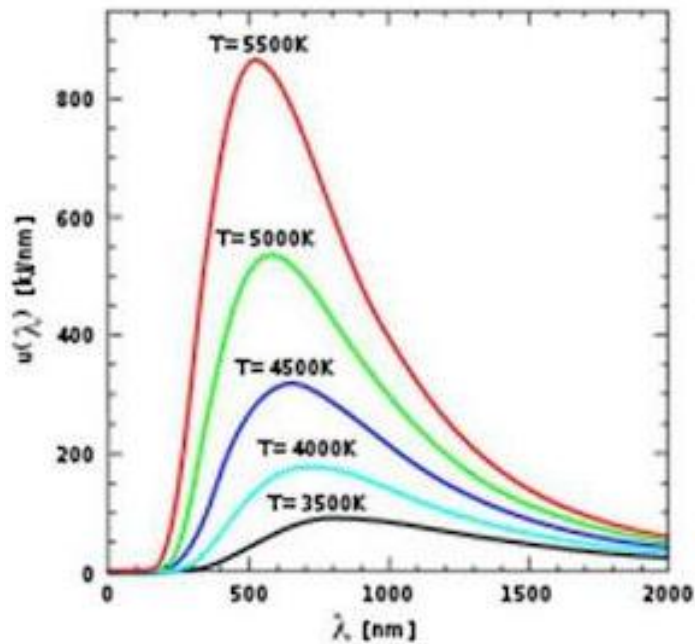
Рис. Зависимость мощности излучения чёрного тела от длины волны (Закон смещения Вина)
