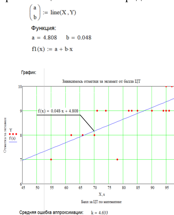
Рис.16. Линейная регрессия
