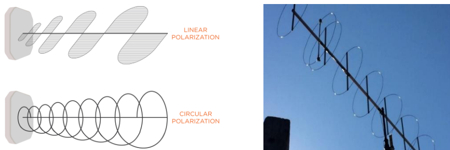
Рис.2. Антенна с круговой поляризацией.
