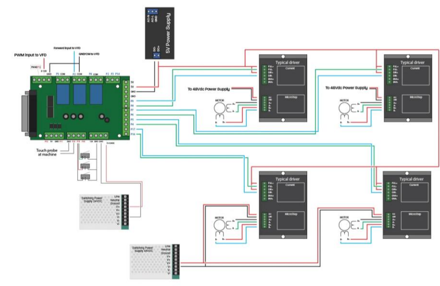
Рис.2. Схема подключения системы ЧПУ Mach3.
