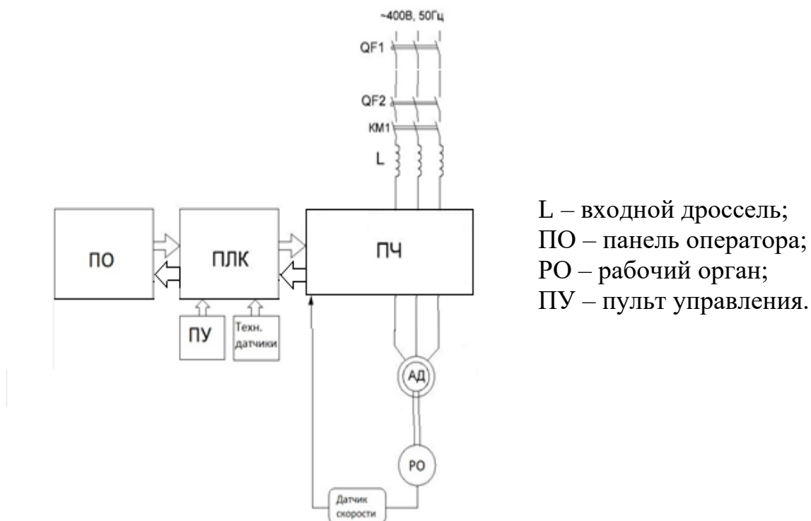
Рис.1. Функциональная схема электропривода.
