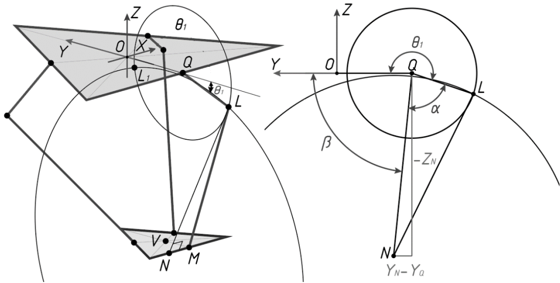
Рис.7 – Геометрические построения для решения задачи обратной кинематики.
