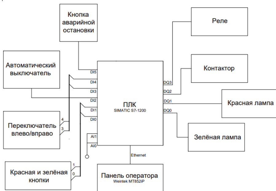
Рис.1. Структурная схема шкафа управления.
