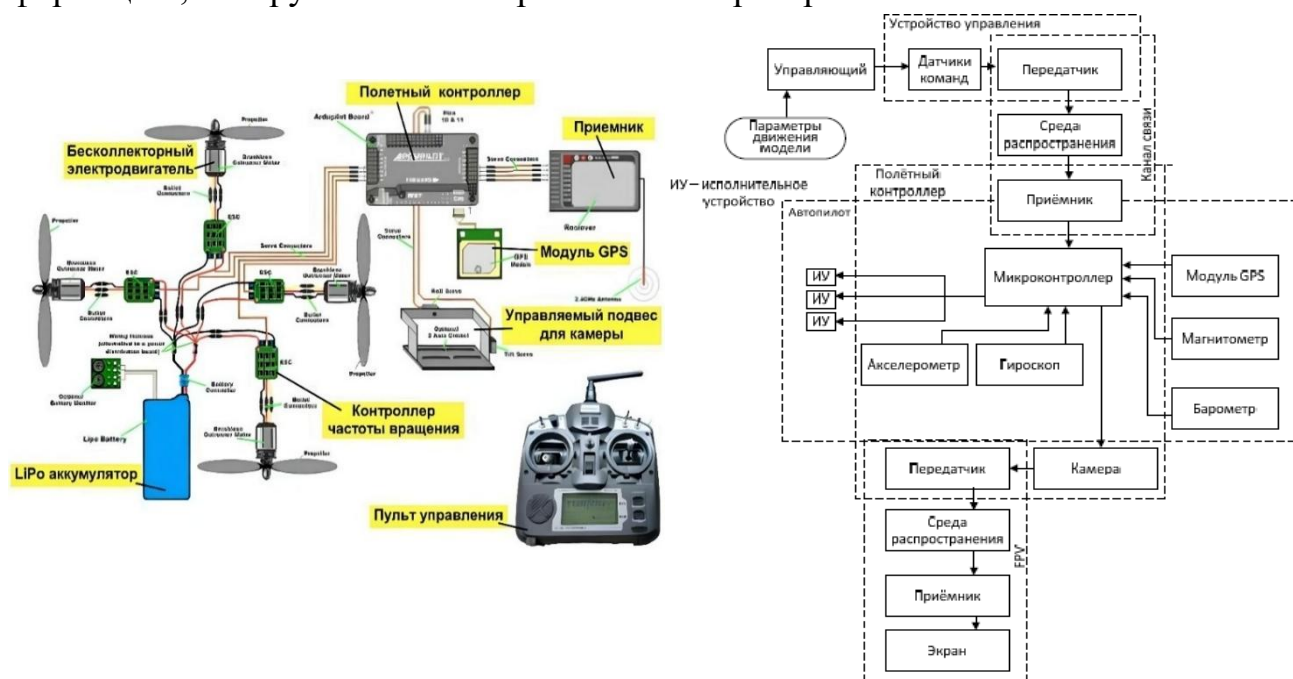
Рис.2. Структурная схема (слева) и алгоритмическая блок-схема (справа) современного беспилотного летательного аппарата (БПЛА).
