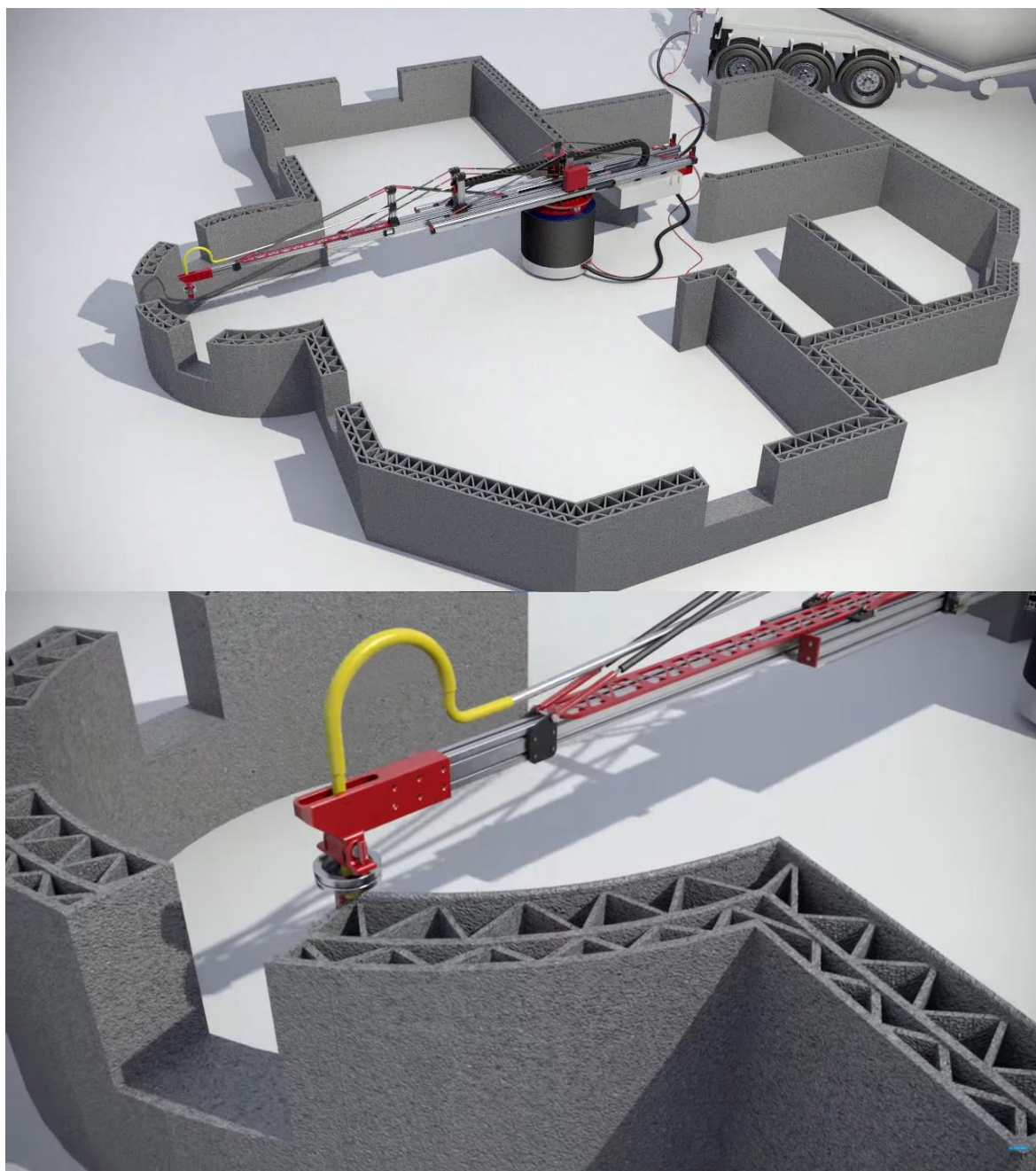
Рис.1. Бетонная 3D-печать.
