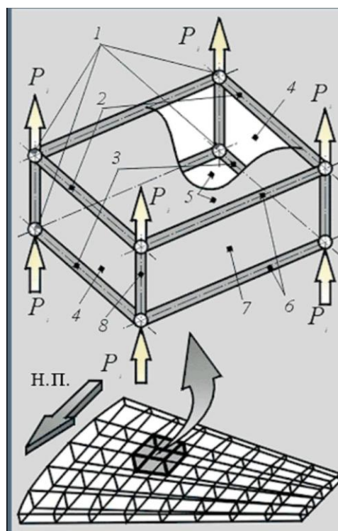
Рис.5. Метод конечных элементов.
