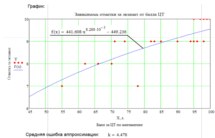
Рис.6. Степенная регрессия.
