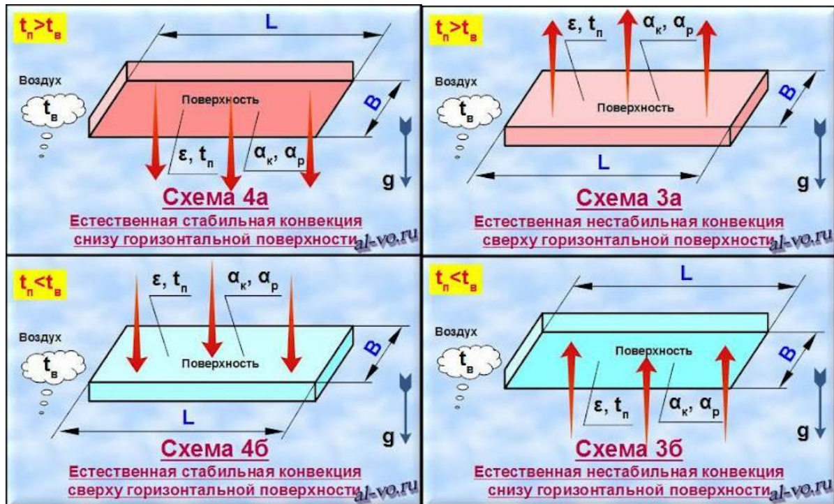
Рис.2. Естественная стабильная и нестабильная конвекции.
