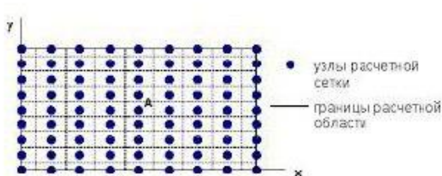
Рис.6. Метод конечных объёмов.
