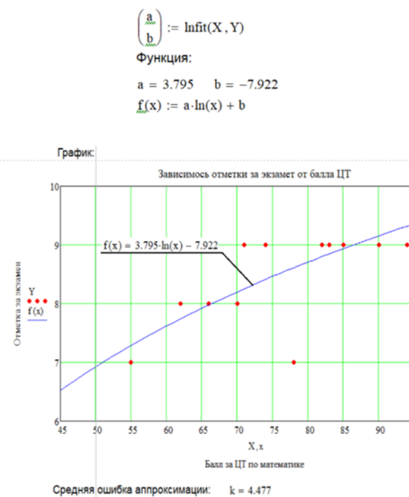
Рис.4. Логарифмическая регрессия.
