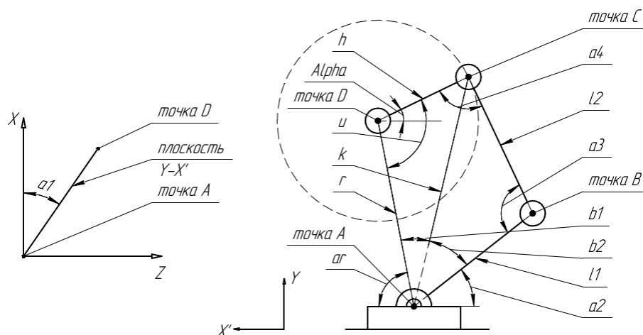
Рис.1. Схема манипулятора.
