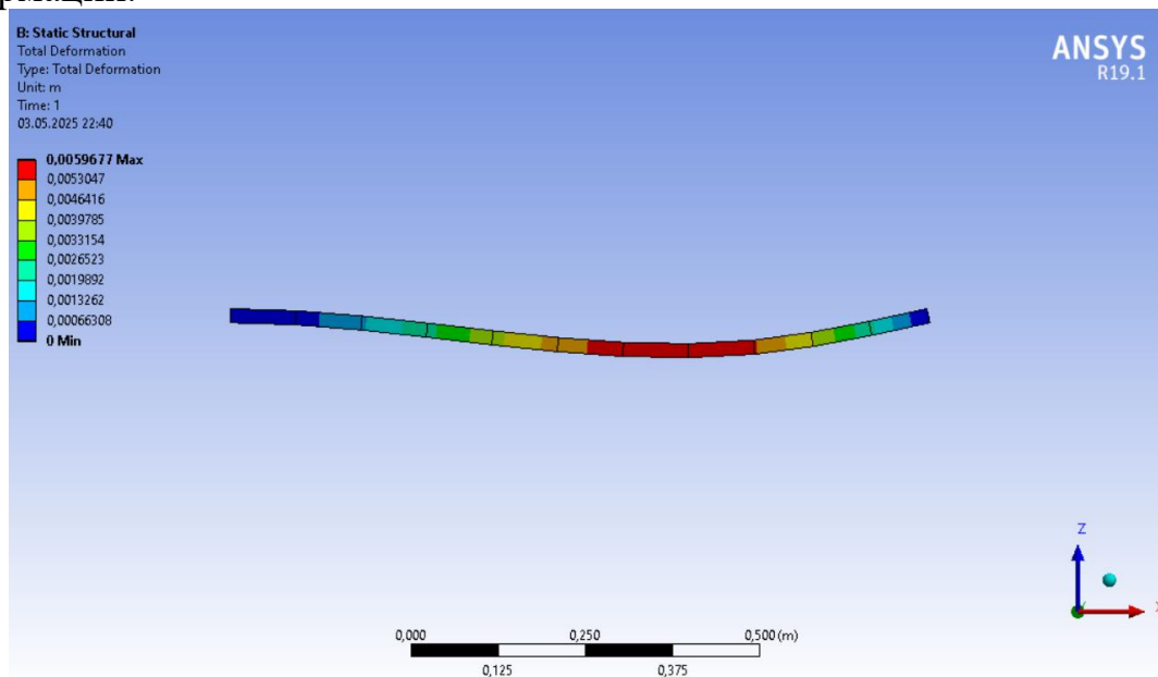
Рис.3. Визуализация деформации балки из DesignModeler.
