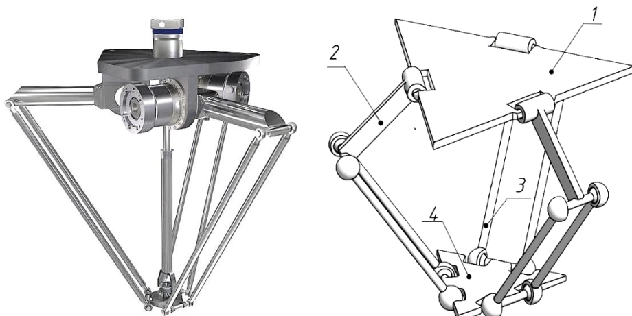
Рис.6. Внешний вид и структурная схема дельта-робота. Обозначения: 1 – основание, 2 – рычаг, 3 – штанга, 4 – платформа
