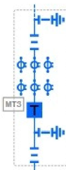
Рис.4. Состояние коммутационных аппаратов до выверки.
