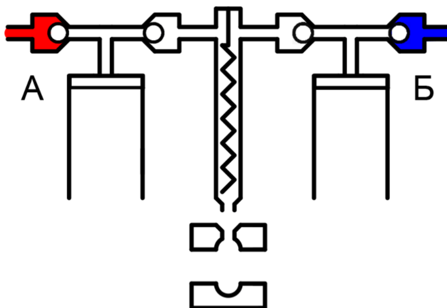
Рис. 1. Функциональная схема станка.
