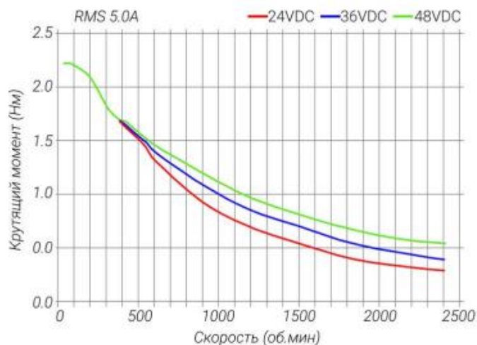
Рис.1. График зависимости момента от скорости шагового двигателя.
