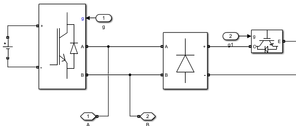
Рис.2. Подсистема силового преобразователя.
