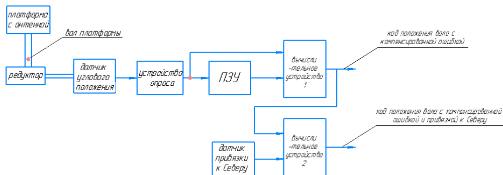
Рис.1. Устройство преобразования углового перемещения антенны.
