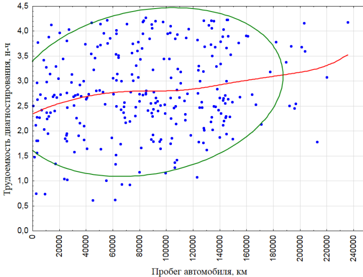
Рисунок 2 – Экспериментальное распределение трудоемкости отдельных диагностических случаев по пробегам автомобиля
