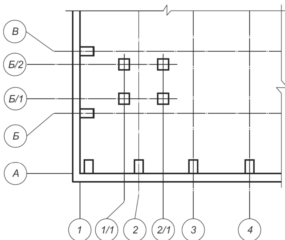
Рисунок 7.3 – Координационные оси
