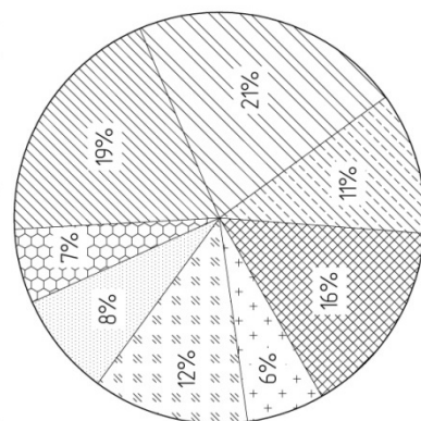
Распределение основных неисправностей стартеров
