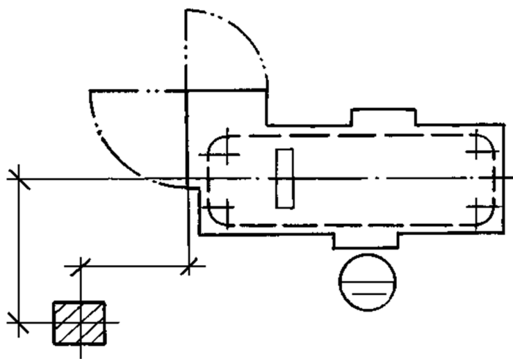
Рисунок 7.4 – Пример привязки оборудования к осям здания
