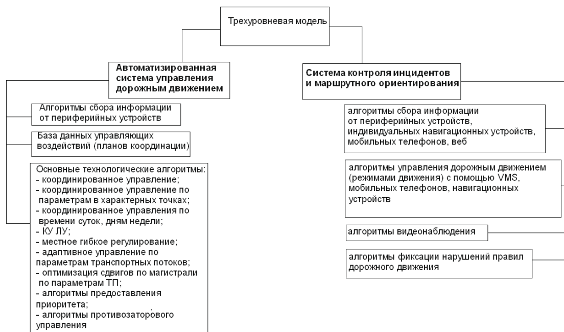
Рисунок 1 – Трехуровневая модель как связующее звено
