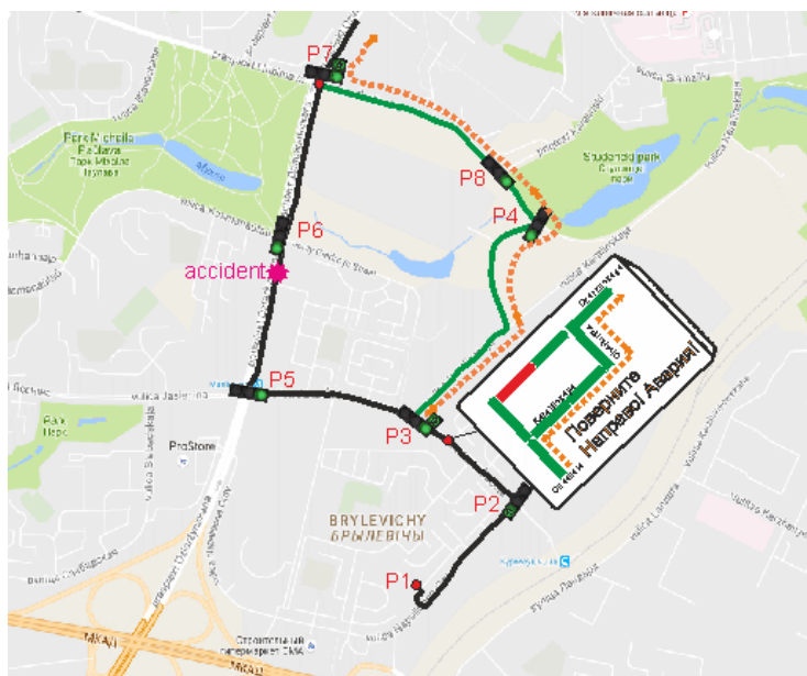
Рисунок 4 – Сценарий с ДТП и использованием водителем кратчайшего пути (маршрут № 1)
