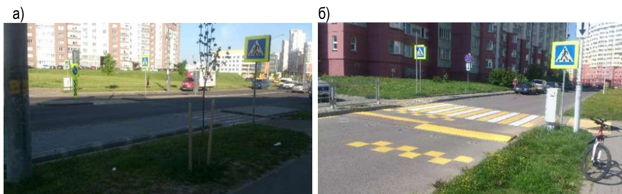
Рисунок 9 – Комбинированное применение сужений проезжей части, искусственных неровностей и светодиодных ламп, установленных у основания искусственной неровности (а – ул. Я. Чечота, 21, г. Минск; б – ул. Я. Чечота, 20, г. Минск)
